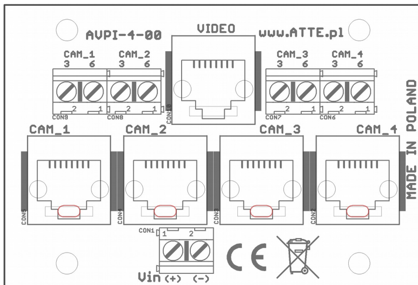
Rys. 1. Widok urządzenia AVPI-4-00-OF
