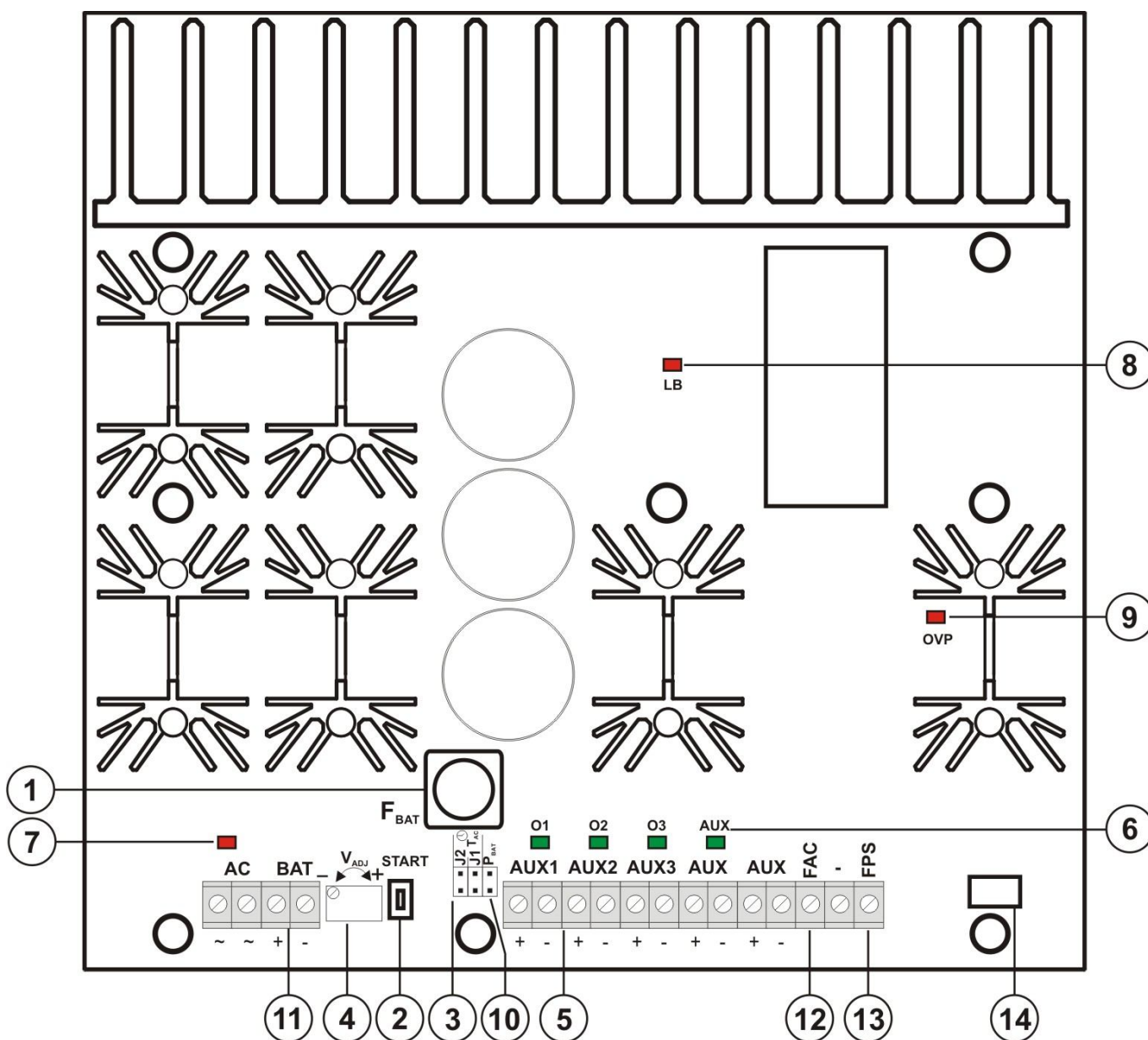
Rys.2. Widok płyty PCB zasilacza.
