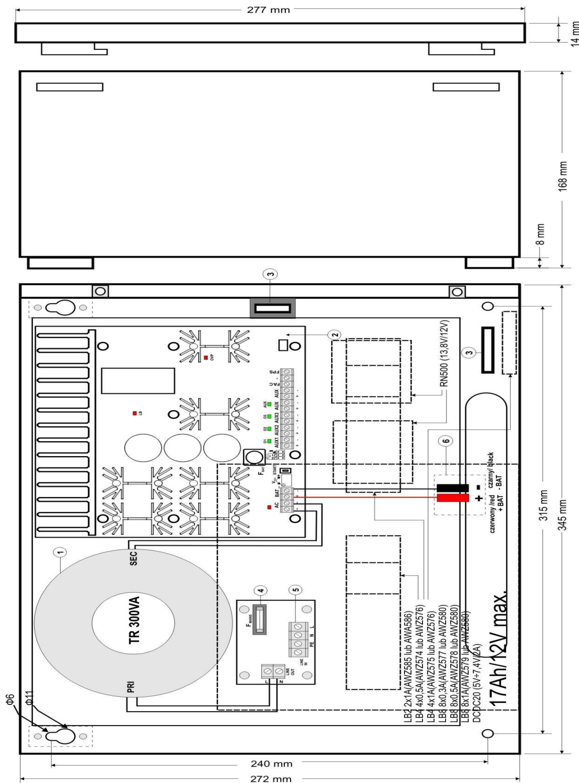
Rys.3. Widok zasilacza.
