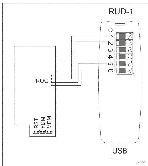
Rys. 4. Podłączenie zamka do interfejsu RUD-1
