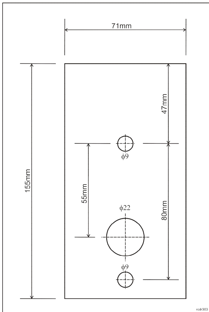
Rys.5 Podkładka dystansowa.
