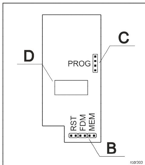
Rys. 2. Moduł elektroniczny w szyldzie zewnętrznym
