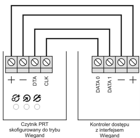
Interfejs Wiegand
