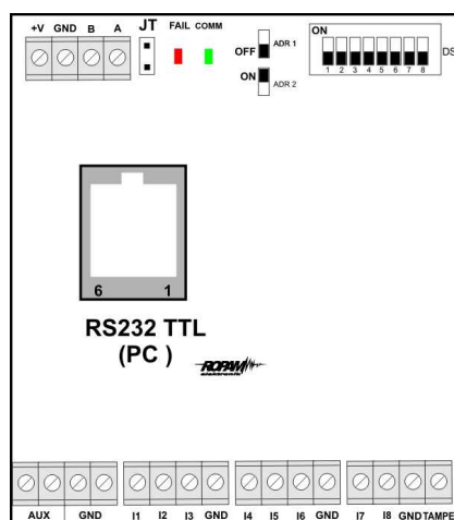
Widok modułu EXP-I8-RN
