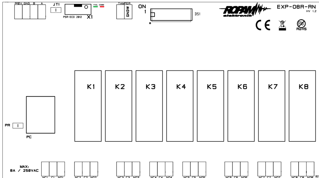
3 Widok modułu EXP-08R-RN
